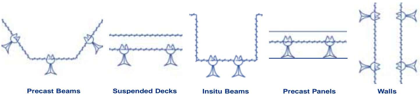
Precast Beams
